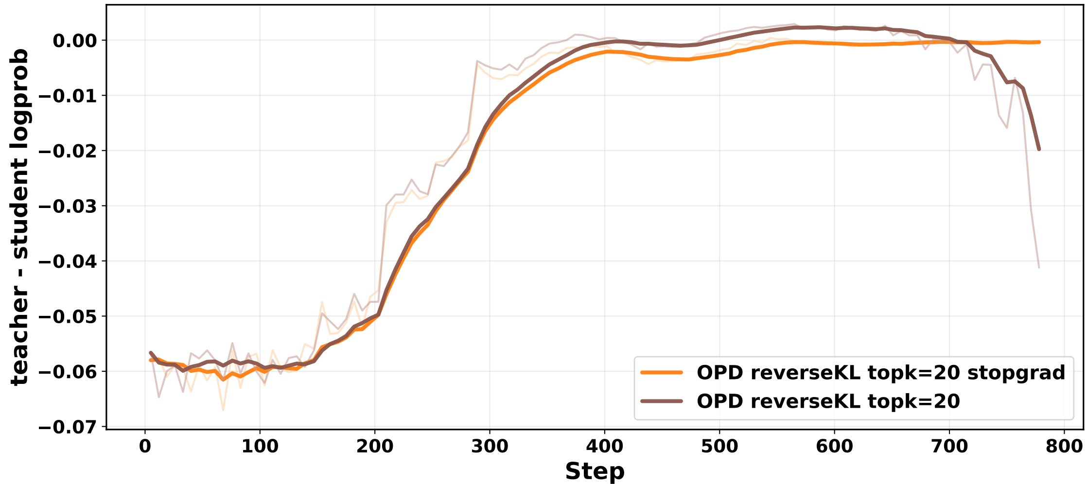
train/other_teacher_minus_student_logprob
